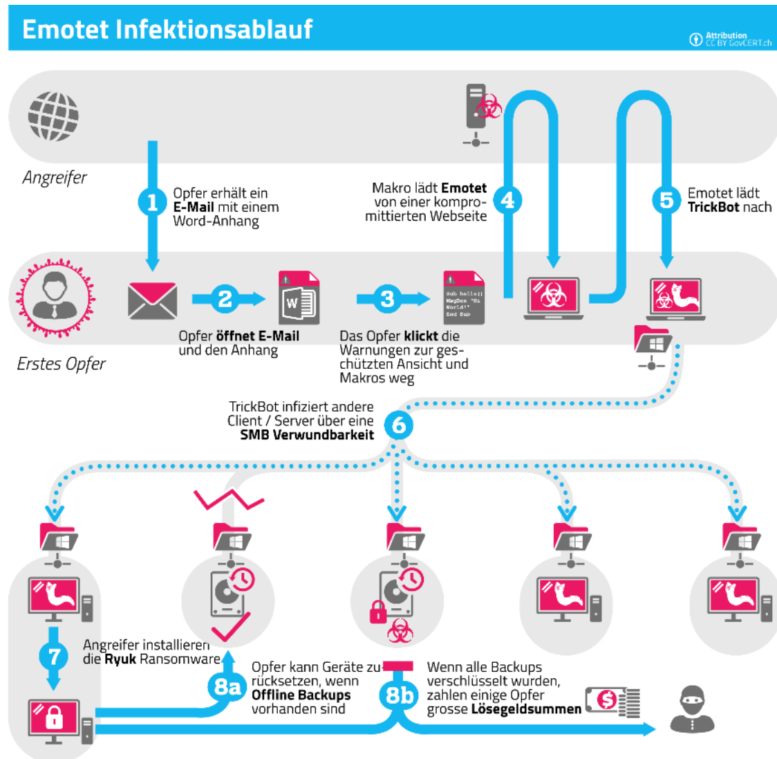
Abb. 2: Emotet Infektionsablauf
